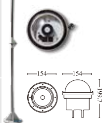
조도수광부(GLX-200)
